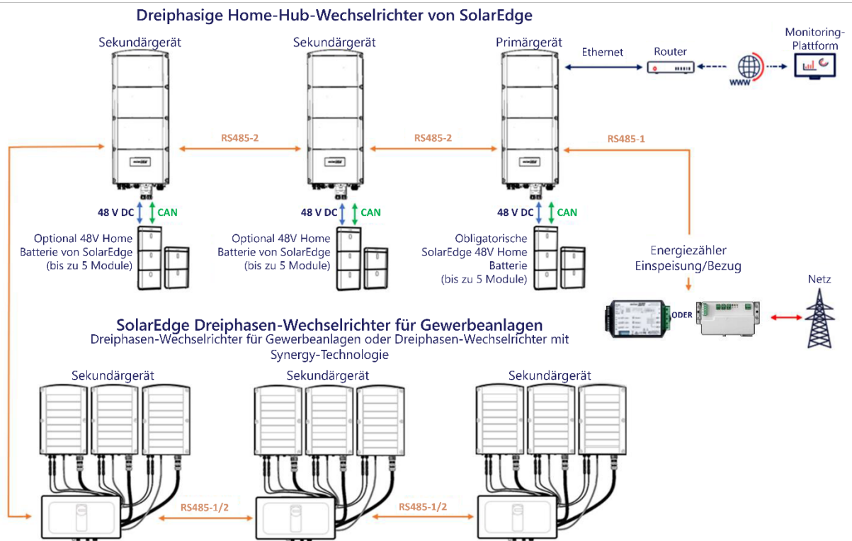
Diagramm eines Gewerbeanlagenspeichers mit einer maximalen Anzahl von Wechselrichtern
