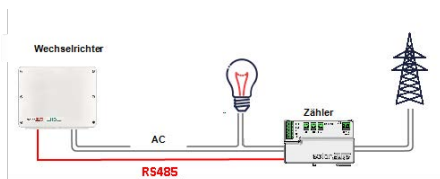
Abbildung 5: Anschluss einzelner Wechselrichter
