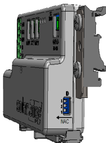
Abbildung 9: Modbus-Adressen- und Terminierungs-DIP-Switches
