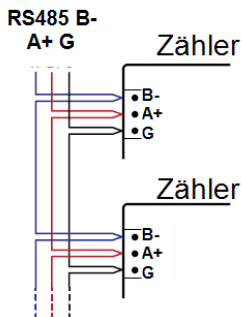
Abbildung 20: RS485-Zählerreihe
