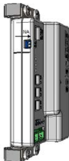
Abbildung 9: Modbus-Adressen- und Terminierungs-DIP-Switches
