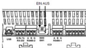
Abbildung 19: RS485-Terminierungs-Switch am Gewerbeanlagen-Gateway
