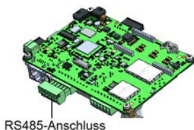
Abbildung 16: RS485-Anschlüsse des Wechselrichters
