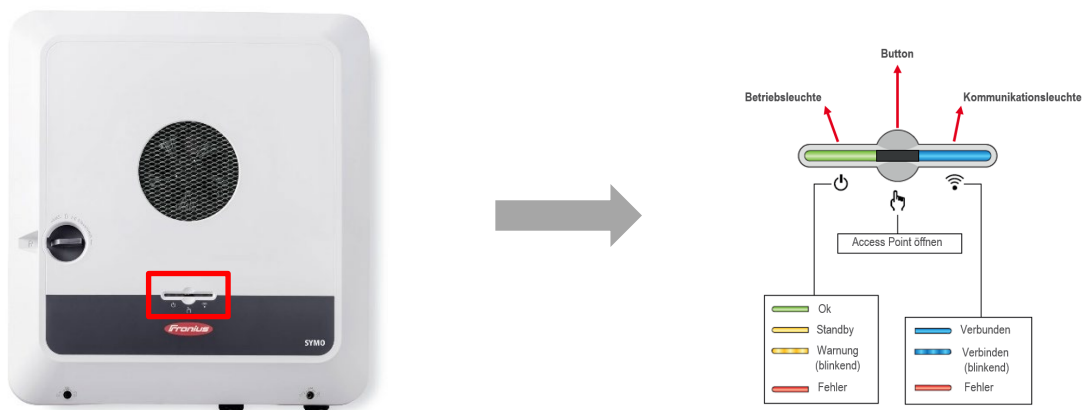
Abbildung 10: Öffnen des lokalen Netzwerkes (Wifi-Access Point) der Fronius GEN24 Plus Wechselrichterserie und Beschreibung der Funktionen der LED-Muster
