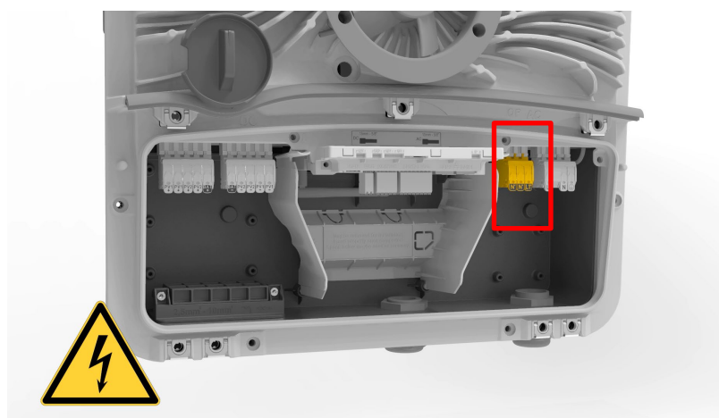
Abbildung 4: Anschlussbereich des Fronius GEN24 Plus mit PV-Point Push-in Federzugklemme
