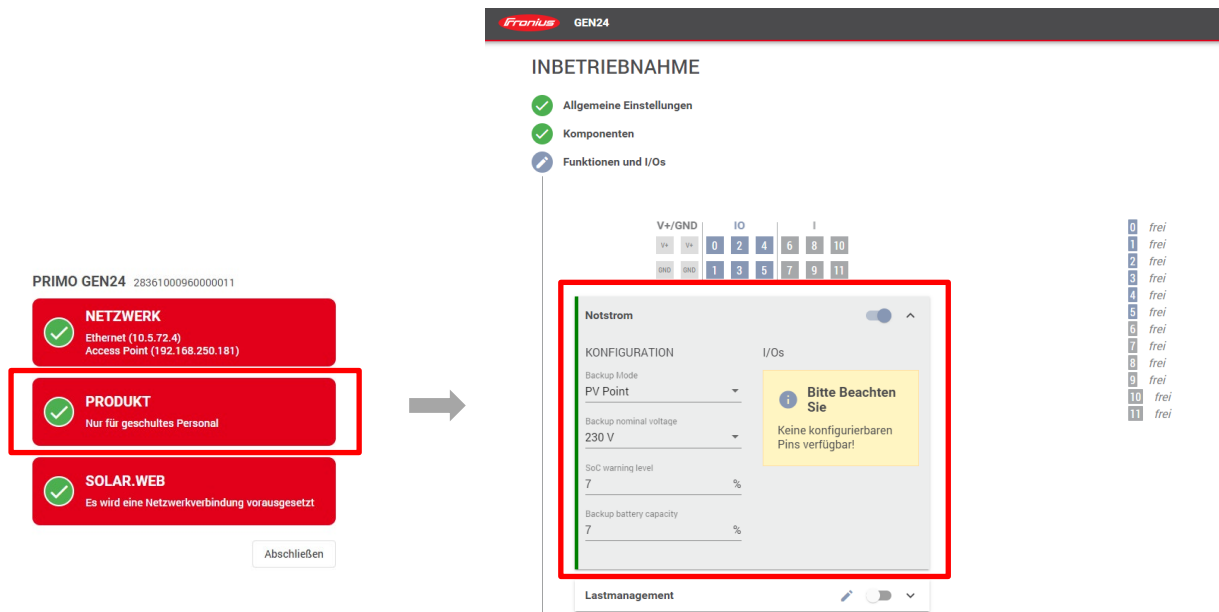
Abbildung 11: Aktivierung des PV-Point im Produkt-Wizard während der Erstinbetriebnahme des GEN24 Plus Wechselrichters
