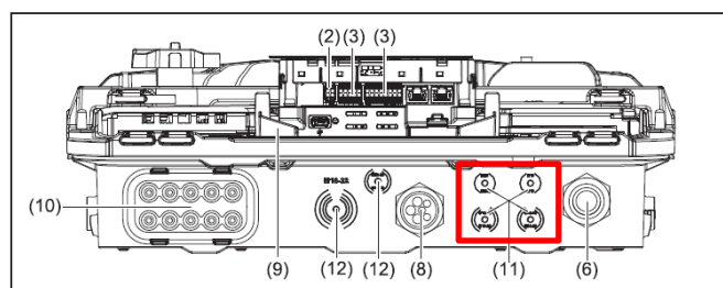
Abbildung 2: Wechselrichter-Unterseite der Fronius GEN24 Plus Serie mit den vier vordefinierten Ausgängen
