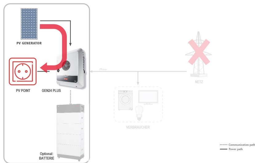
Abbildung 1: Schema der Basis-Notstromversorgung (PV-Point) der Fronius GEN24 Plus Serie
