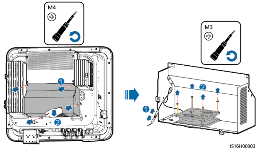
Abbildung 8-1 Entfernen eines fehlerhaften Lüfters
