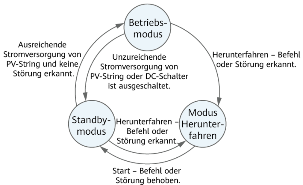
Abbildung 2-9 Arbeitsmodi
