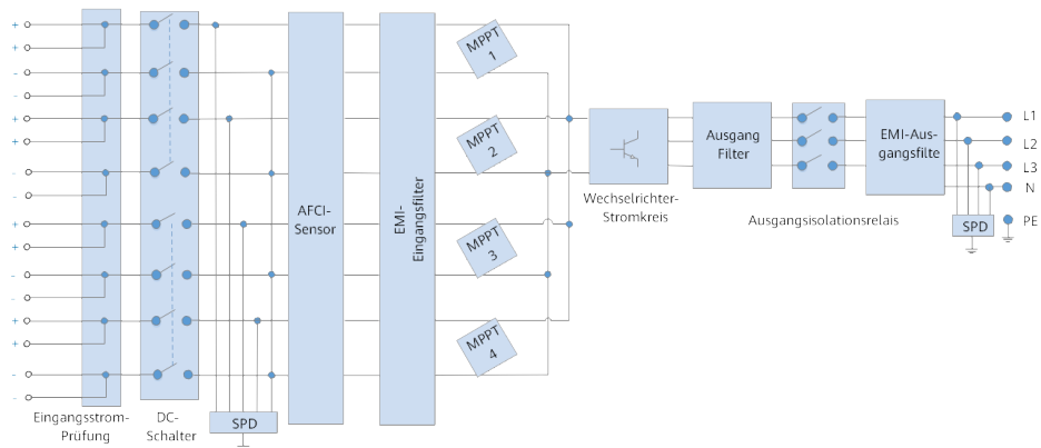
Abbildung 2-8 Schematisches Diagramm
