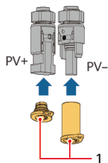
Abbildung 5-22 Verschlussstopfen
