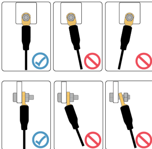
Abbildung 5-11 Verdrahtungsanforderungen
