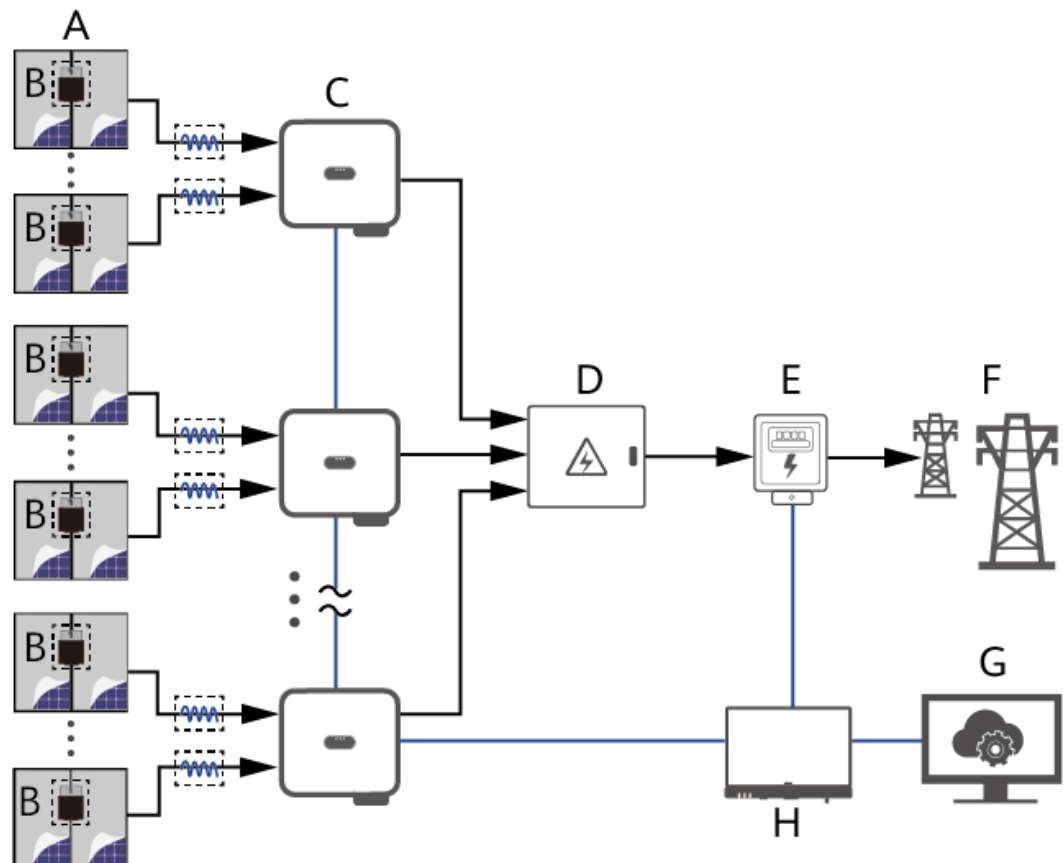
Abbildung 2-2 RS485-Vernetzung (SmartLogger)
