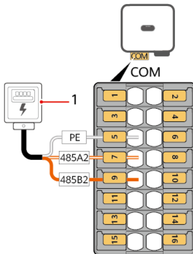
Abbildung 5-36 Kabelverbindung
