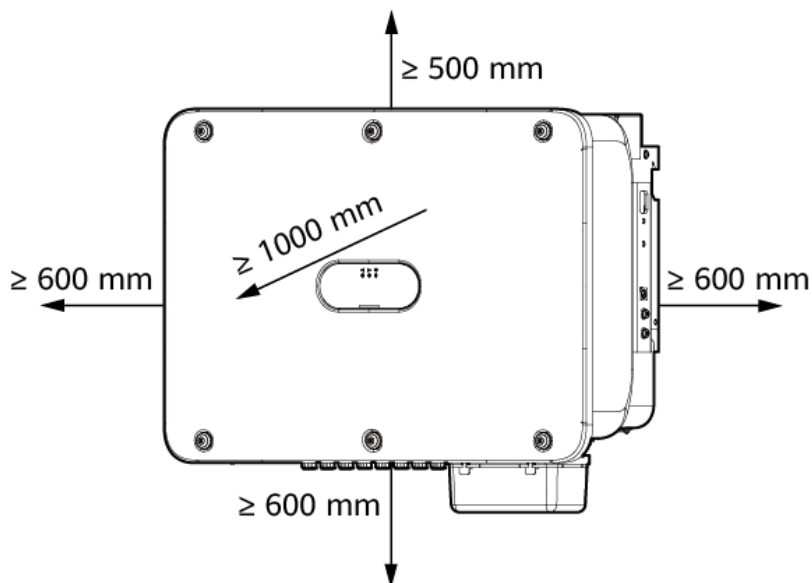
Abbildung 4-3 Abstände
