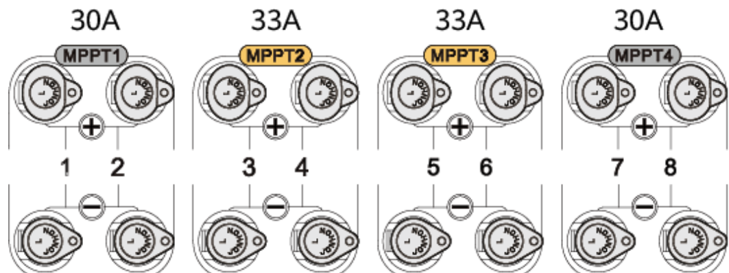
Abbildung 5-12 DC-Eingangsklemmen
