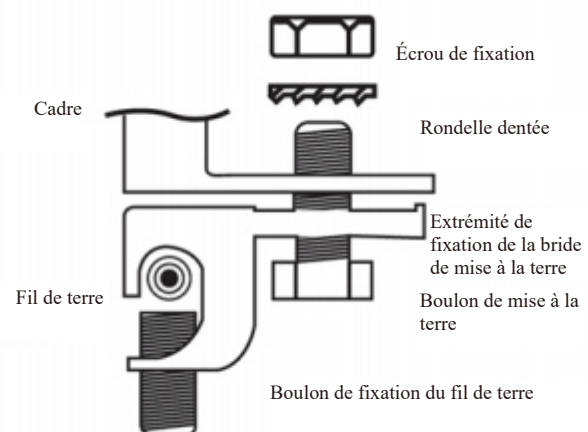
Figure 10 Méthode de mise à la terre par boulon du module photovoltaïque
