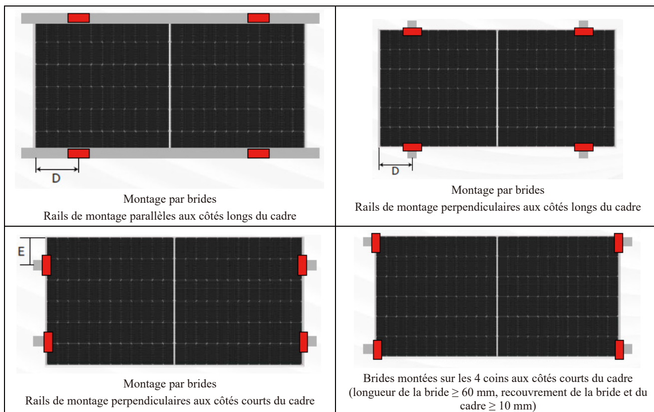
Figure 8 Position d'installation des modules bifaciaux
