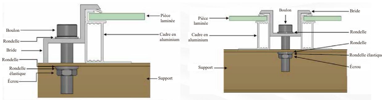
Figure 6 Installation par brides des modules monofaciaux
