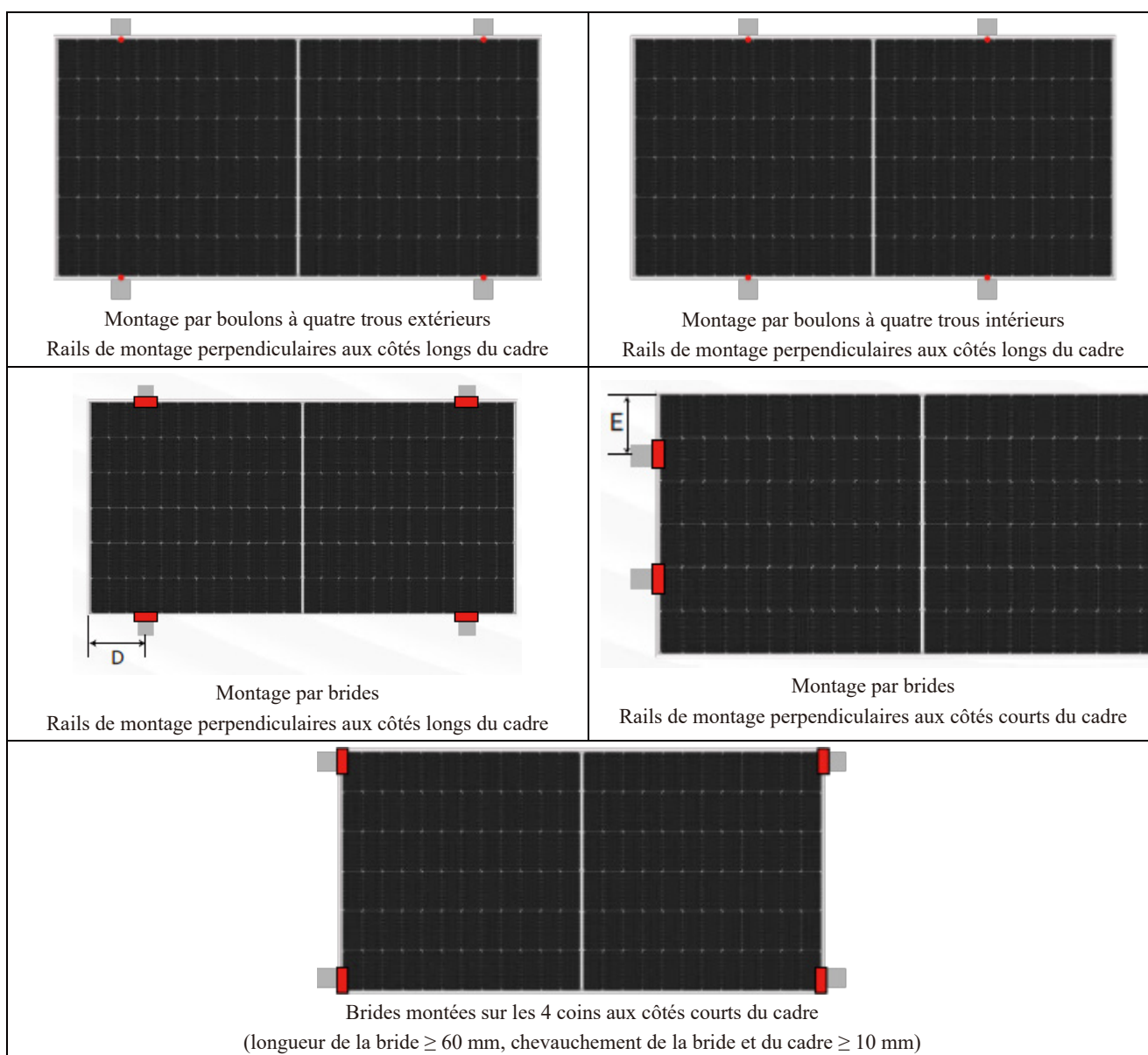
Figure 7 Position d'installation des modules monofaciaux
