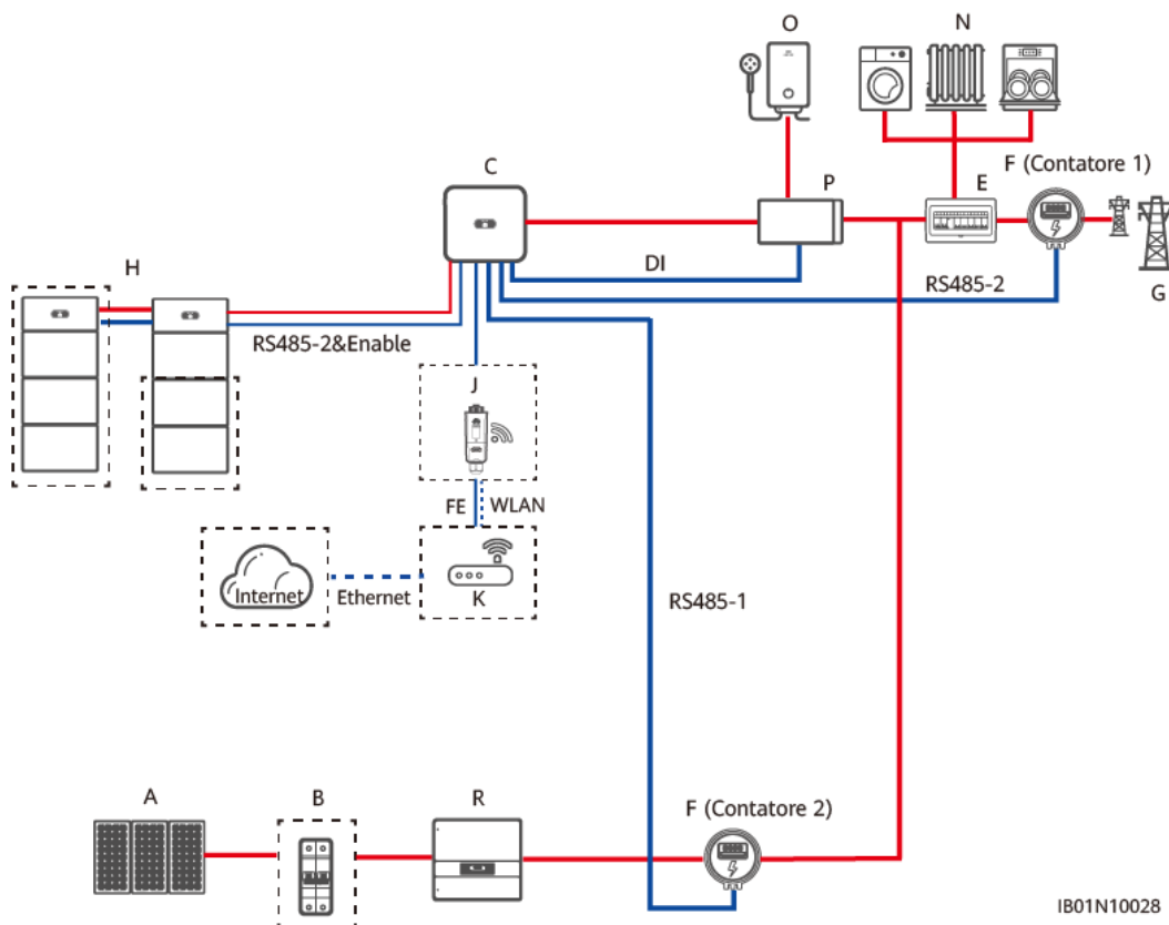
Figura 4-18 Connessione in rete con inverter di terze parti
