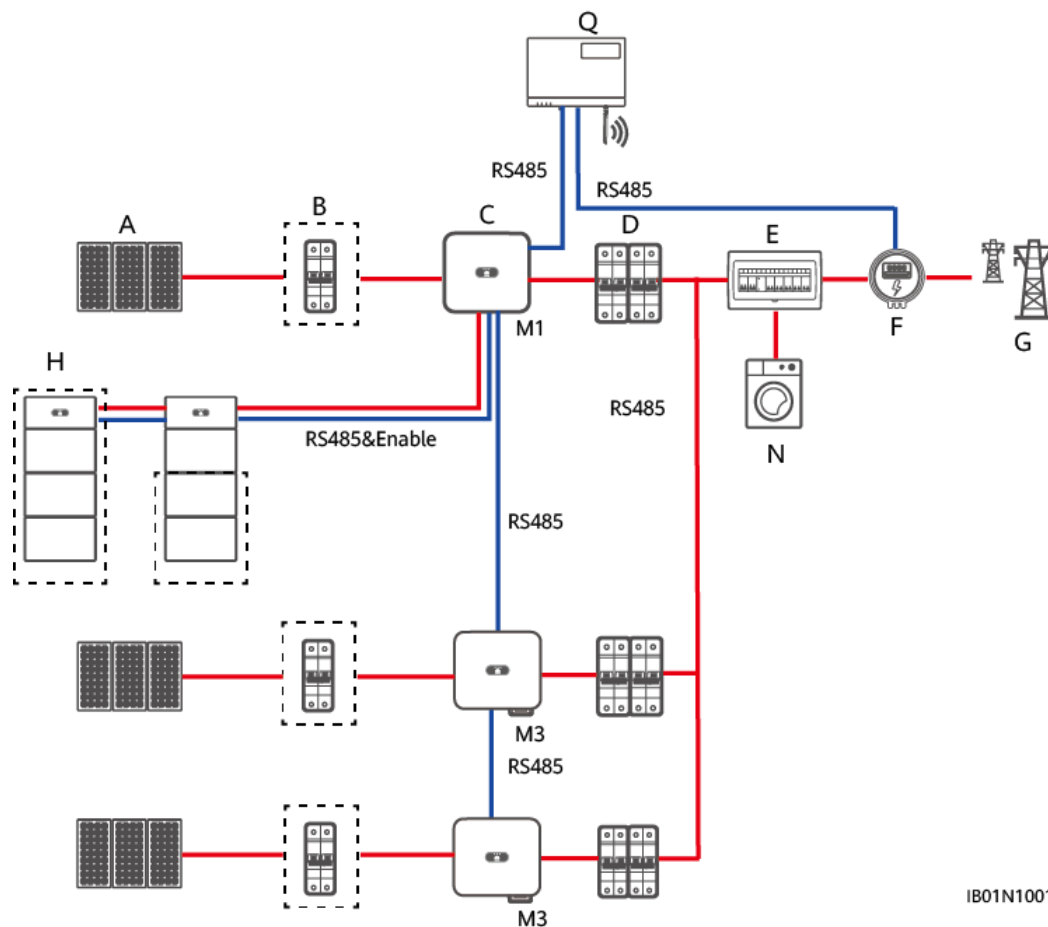
Figura 4-2 Collegamento in rete di un SUN2000-(3KTL-10KTL)-M1 e due SUN2000-(20KTL, 29.9KTL, 30KTL, 36KTL, 40KTL)-M3 (i riquadri tratteggiati indicano i componenti opzionali)
