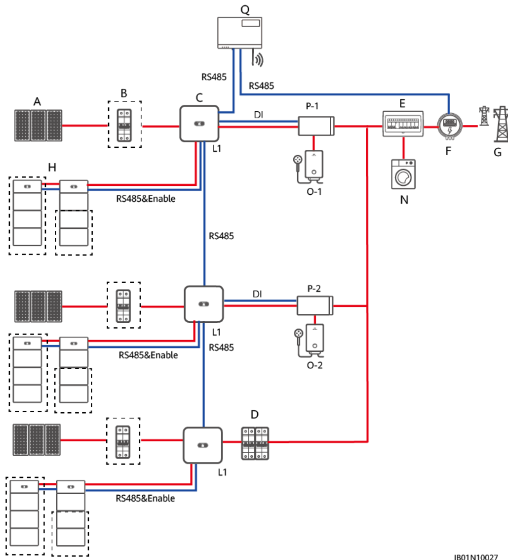
Figura 4-13 Diagramma di connessione di rete degli inverter SUN2000-(2KTL-6KTL)-L1 collegati in cascata (i riquadri tratteggiati indicano i componenti opzionali)
