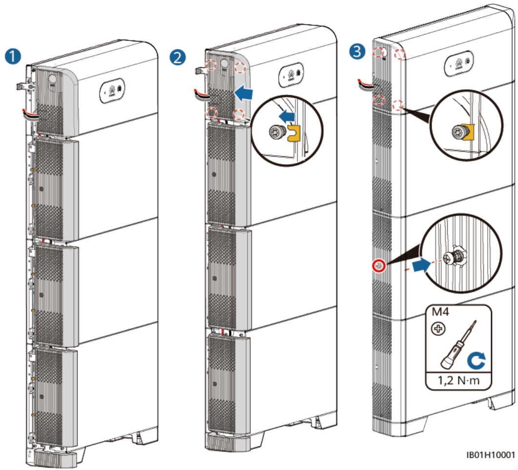
Figura 6-17 Installazione del coperchio
