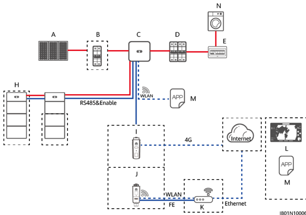
Figura 4-16 ESS non in rete (i riquadri tratteggiati indicano i componenti opzionali)
