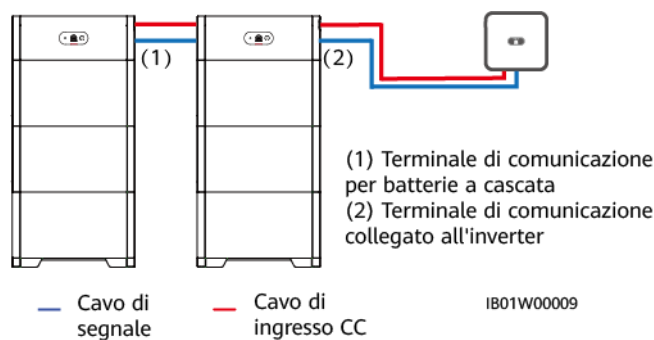
Figura 6-14 Connessione dei cavi per collegamento in cascata delle batterie
