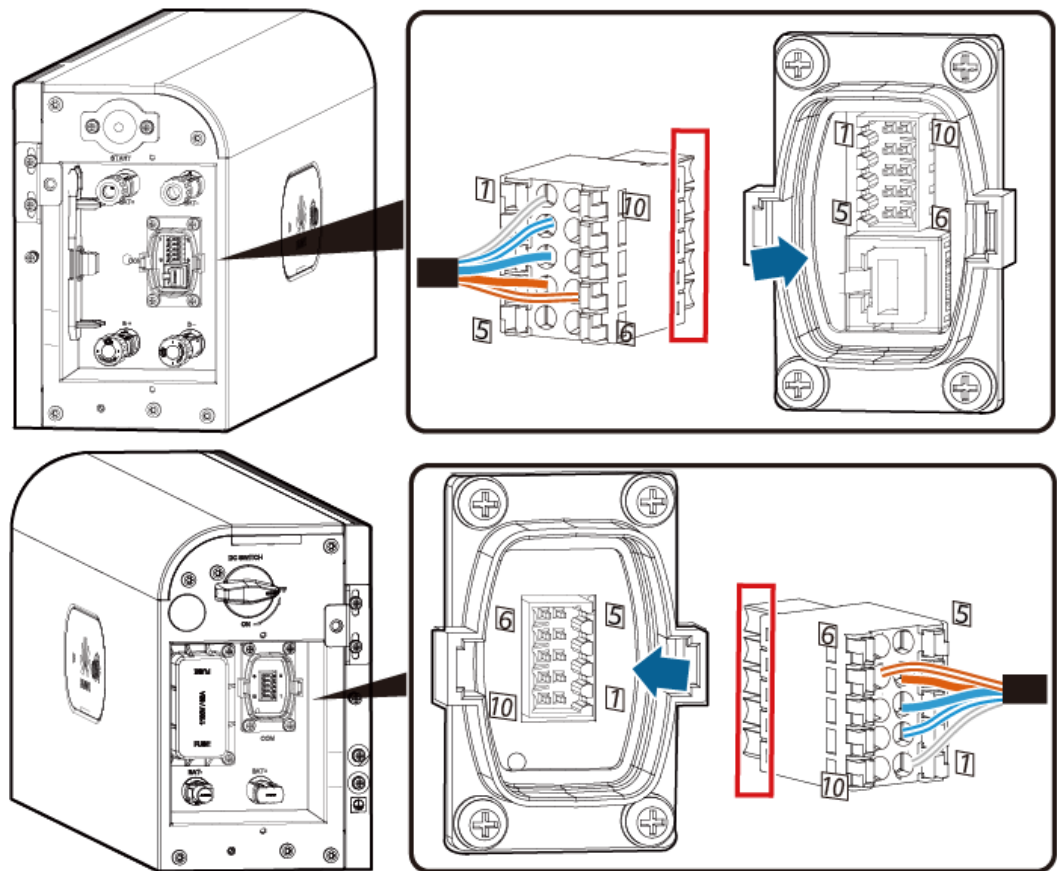
Figura 6-12 Inserimento del terminale
