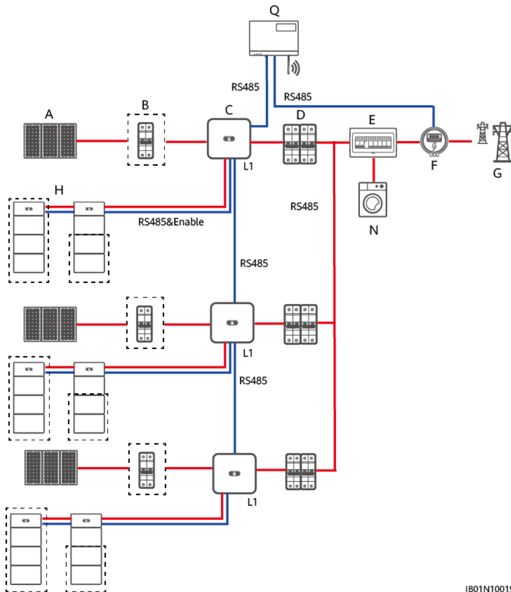
Figura 4-3 Diagramma di connessione di rete degli inverter SUN2000-(2KTL-6KTL)-L1 collegati in cascata (i riquadri tratteggiati indicano i componenti opzionali)
