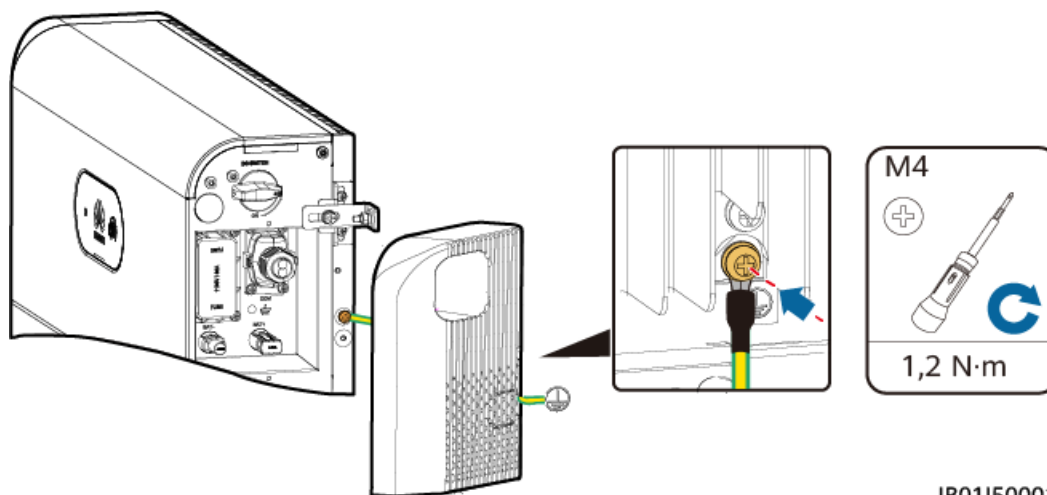
Figura 6-8 Messa a terra del cavo PE
