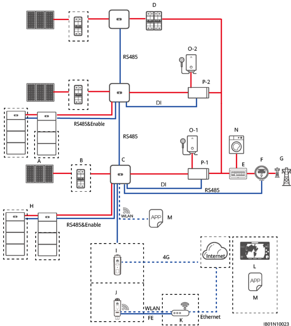
Figura 4-14 Connessione in rete dello Smart Dongle in un ESS collegato alla rete e non in rete (i riquadri tratteggiati indicano i componenti opzionali)
