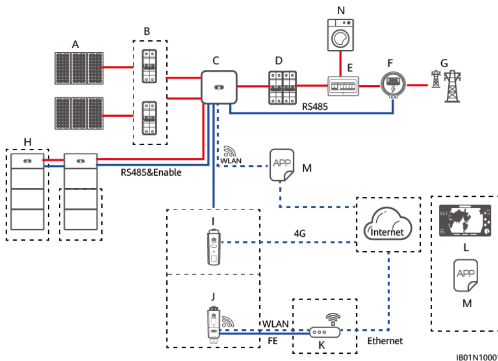
Figura 4-1 Diagramma di connessione in rete di un ESS collegato alla rete (i riquadri tratteggiati indicano i componenti opzionali)
