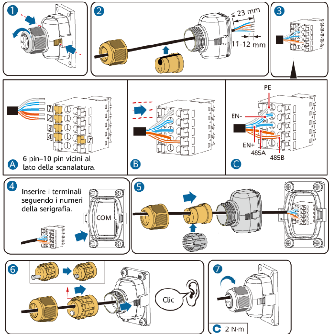
Figura 6-13 Collegamento dei terminali dell'inverter
