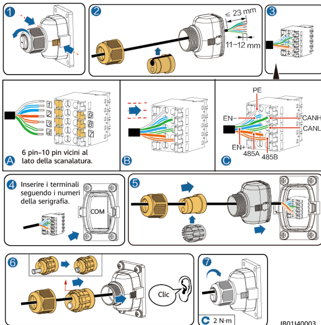
Figura 6-16 Terminale di comunicazione per collegamento in cascata
