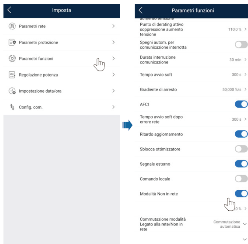
Figura 4-15 Impostazione dell'alimentazione backup
