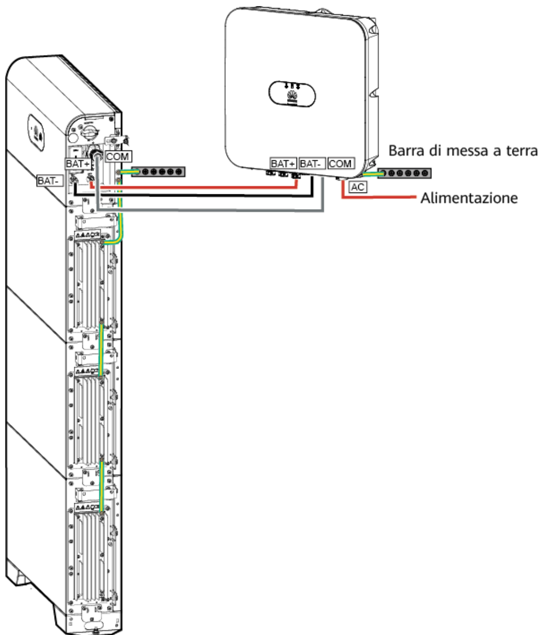
Figura 8-3 Schema di collegamento dei cavi
