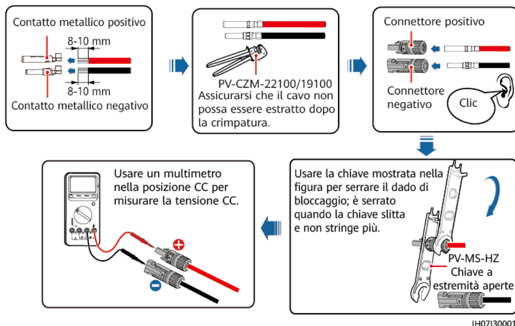
Figura 6-9 Assemblaggio dei connettori CC
