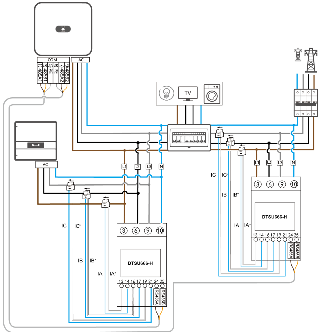
Figura 4-20 Collegamenti dei cavi del contatore elettrico per SUN2000-(3KTL-10KTL)-M1
