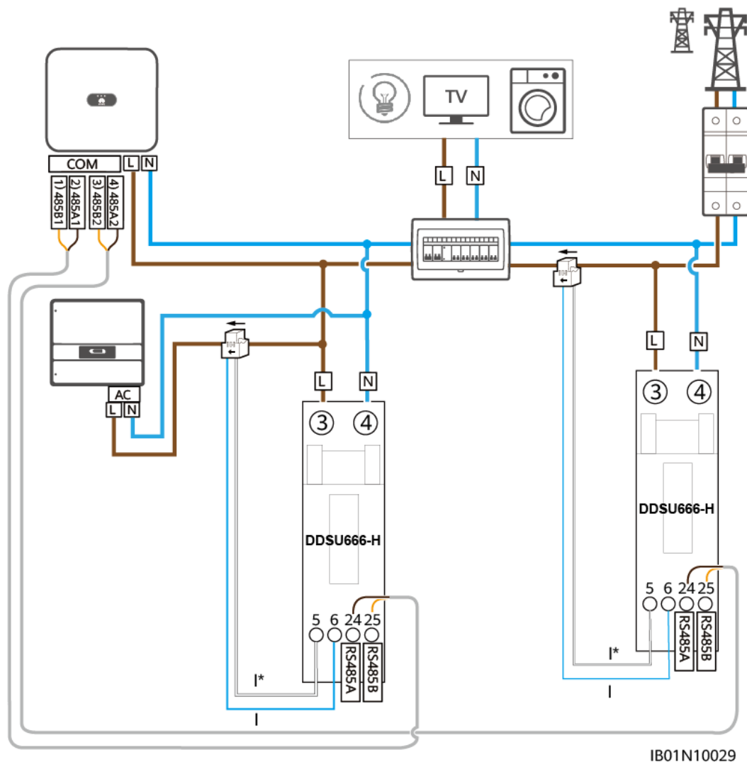
Figura 4-19 Collegamenti dei cavi del contatore elettrico per SUN2000-(2KTL-6KTL)-L1
