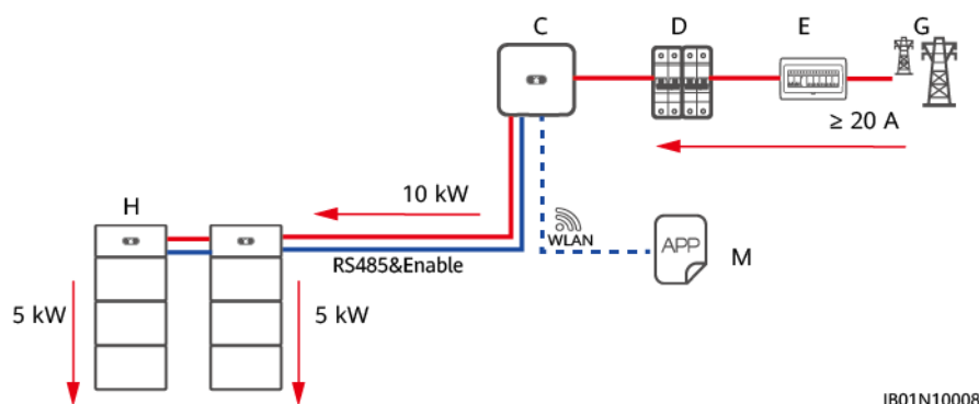
Figura 8-1 Diagramma di rete per uno scenario con alimentazione trifase
