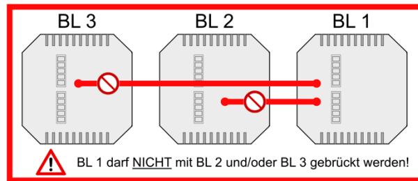
Figura 16: Caricabatterie 1, 2 e 3 Lato posteriore
