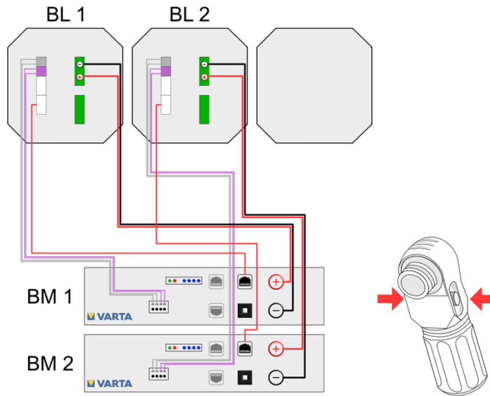
Figura 6: Caricabatterie 1 e 2, modulo batteria 1 e 2
