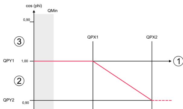
Figura 10: curva caratteristica Q(P)
