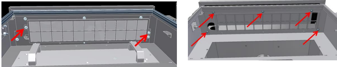
Figura 17: smontaggio filtro dell'aria (vista anteriore dal basso)
