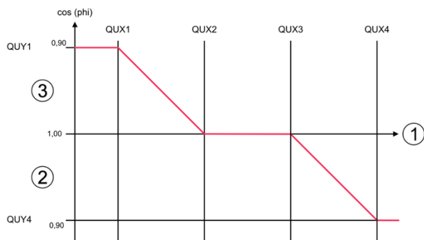
Figura 11: curva caratteristica Q(U)
