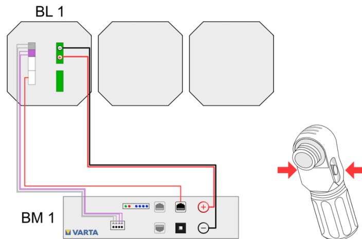
Figura 4: Caricabatterie 1 - Modulo batteria 1
