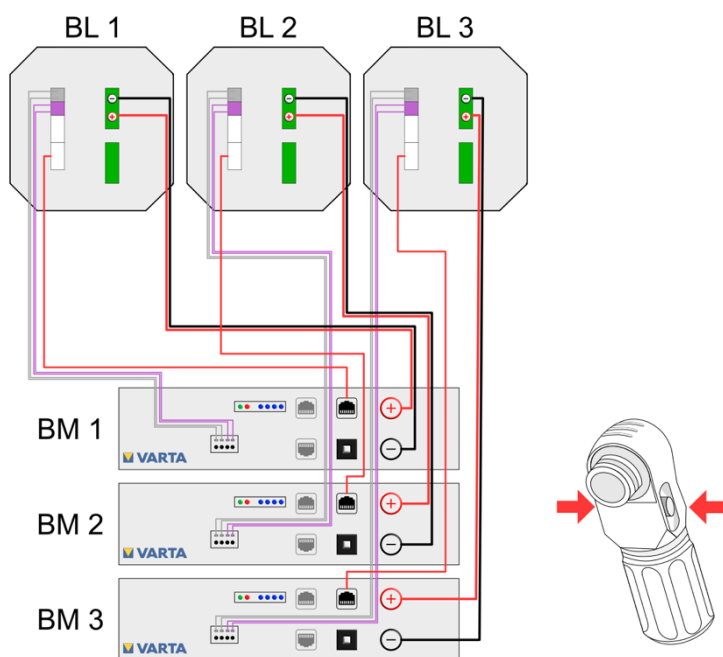
Figura 8: Caricabatterie 1 e 2, moduli batteria 1, 2 e 3,
